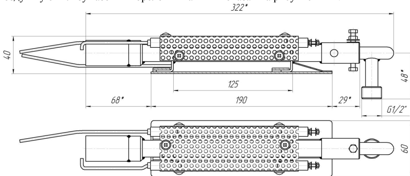
Рисунок 1. Габаритные и присоединительные размеры горелки ПГ-28М:
