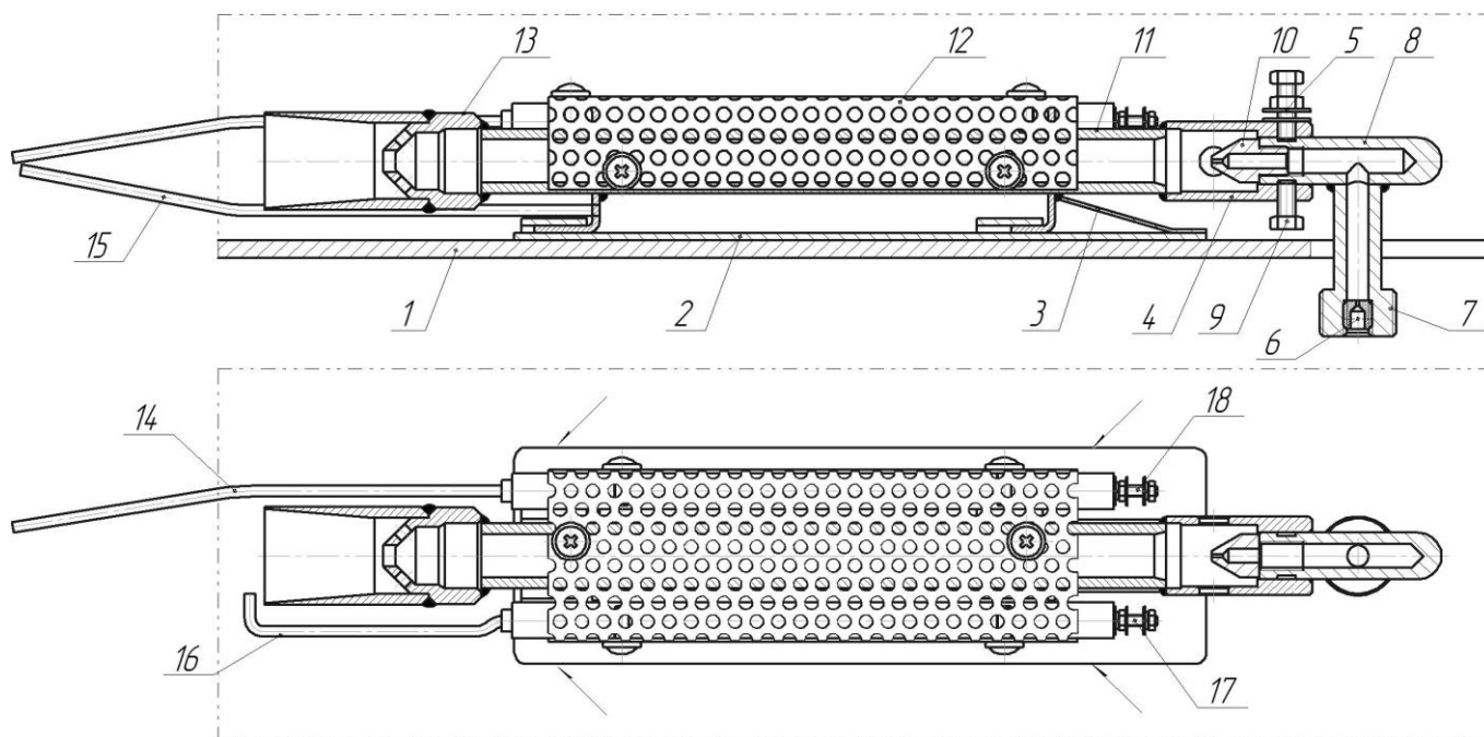
Рисунок 2. Общий вид горелки ПГ-28М:
